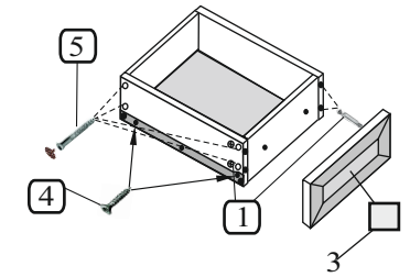
Схема сборки ящика
