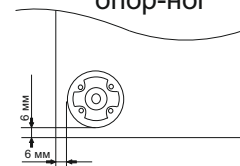
Схема присадки опор-ног
