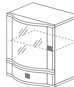
Антресоль КМ - 215 720*540*365
