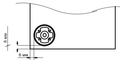
Схема присадки опор-ног
